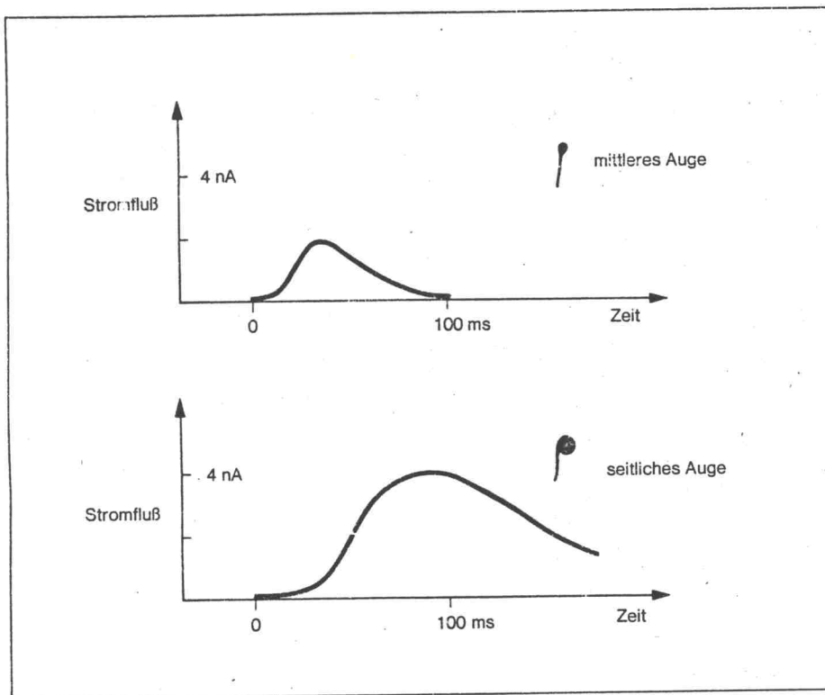
Bild 3: Blitzlicht-induzierter Stromfluß im optischen Nerv der Seepocke. Die Blitzdauer war 10\mu\text{s} . Man beachte, daß für das mittlere Auge (oben) die Geschwindigkeit des Ablaufs größer und die Höhe des Stromes kleiner ist als für das seitliche Auge (unten).
